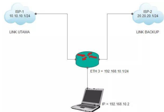
Gambar 1. Failover dan Load balance
