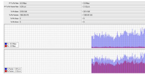
Gambar 8. Grafik Koneksi Link Backup
